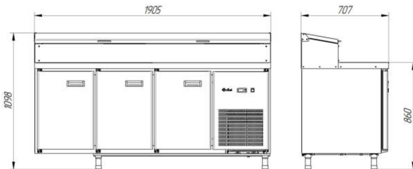
Рис.7. Габаритные размеры СХС-70-02-П столешница с бортом (дверь, дверь, дверь)*
