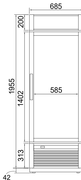
ВИД СПЕРЕДИ
