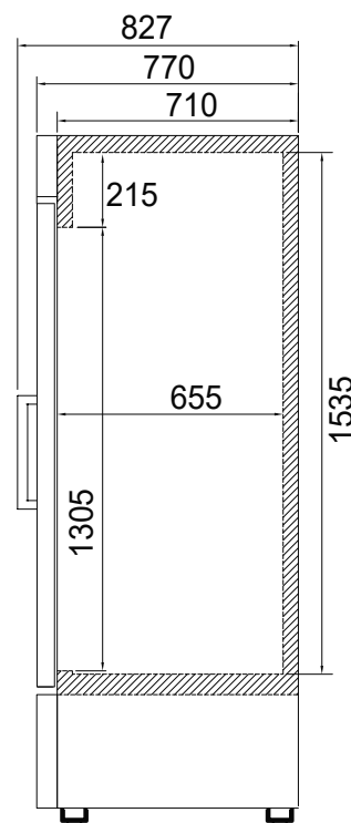
ВИД СБОКУ
