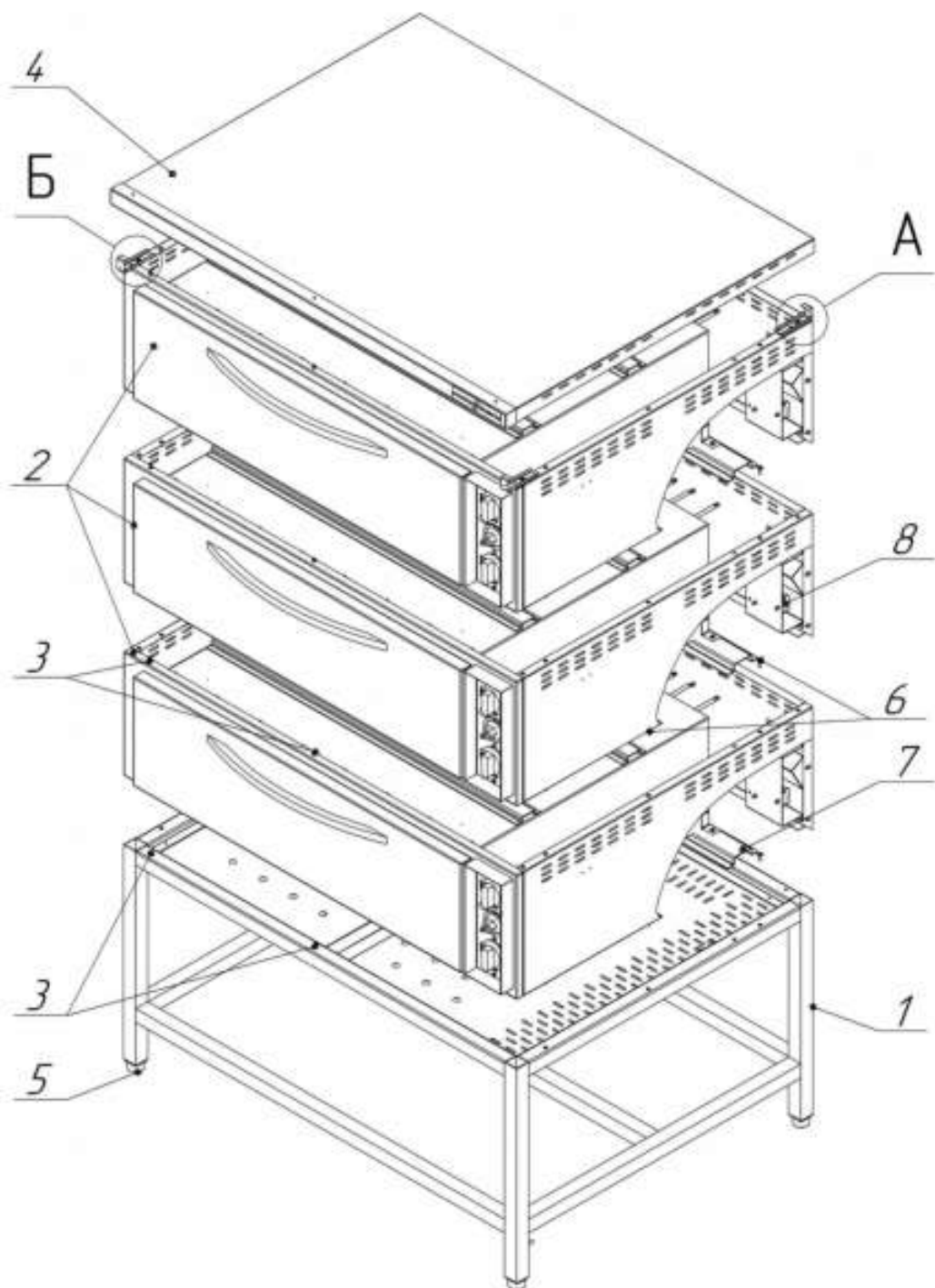
Рисунок 3. Схема сборки
