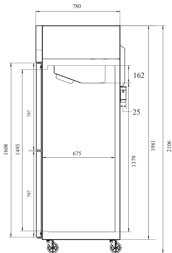
ВИД СБОКУ
