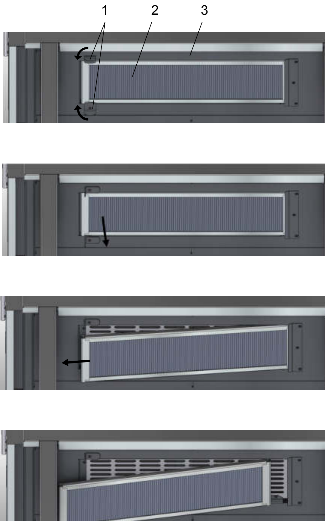
Рис. 5. Извлечение жировулавливающего фильтра.
