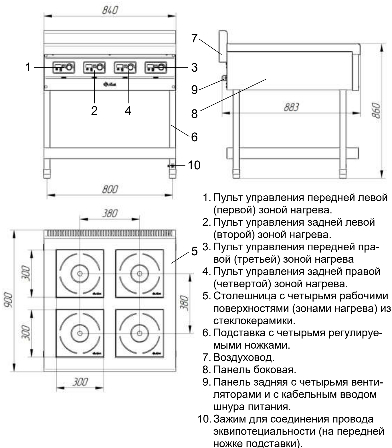
Рис. 2. Общий вид и размеры плит КИП-49П-3,5, КИП-49П-3,5-01, КИП-49П-5,0, КИП-49П-5,0-01
