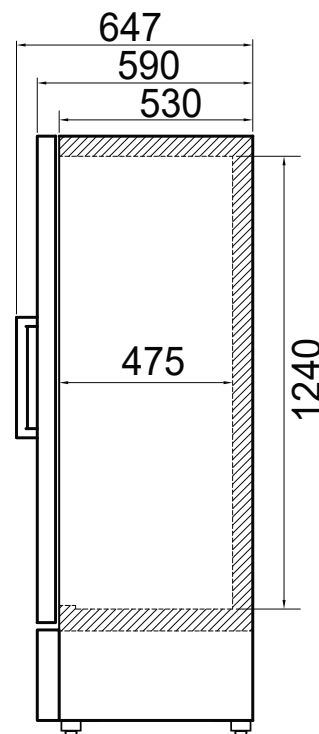
ВИД СБОКУ
