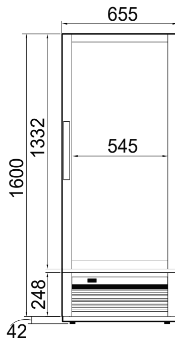
ВИД СПЕРЕДИ
