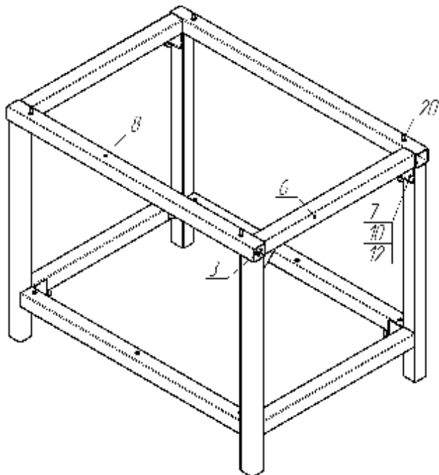
Рисунок 9. Сборка верхней части подставки
