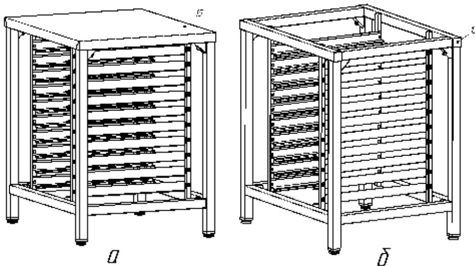
Рисунок 7. Завершение сборки
