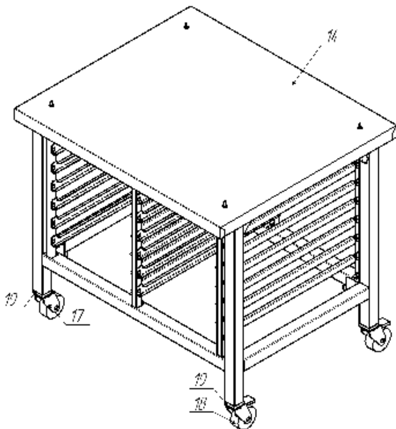
Рисунок 11. Завершение сборки
