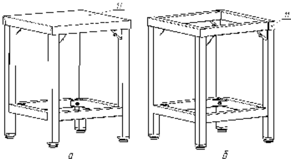
Рисунок 3. Завершение сборки
