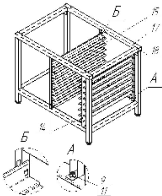
Рисунок 21. Завершение сборки
