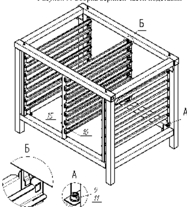
Рисунок 10. Установка стоек направляющих и навешивание направляющих
