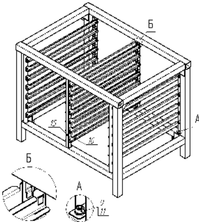
Рисунок 17. Установка стоек направляющих и навешивание направляющих
