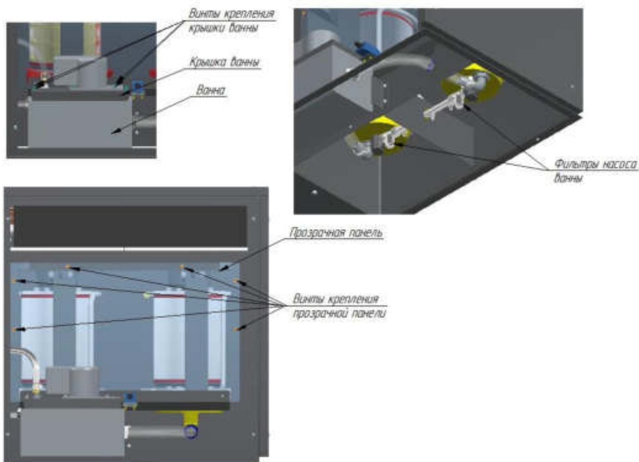
Рис. 9 Расположение крышки ванны, фильтра насоса и прозрачной панели. Смотровая панель на рис. 9 не показана.
