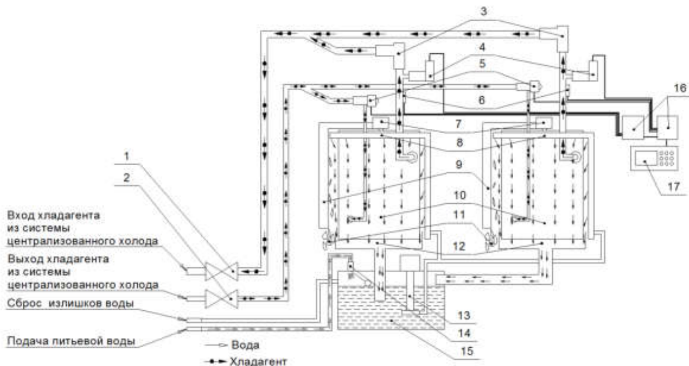
Рис.4 Режим заморозки
