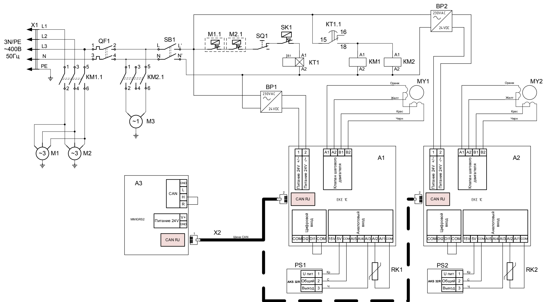
Рис 12. Схема электрическая соединений ЛГ-1200Ч-03.
