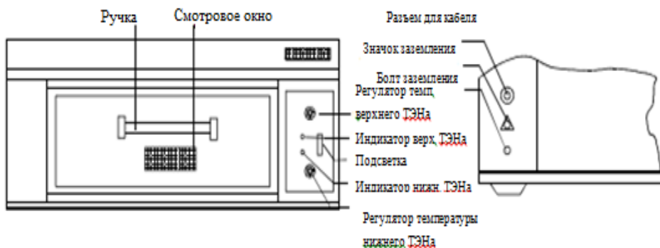
Рис1. Схематическое исполнение передней панели печи
