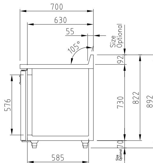
ВИД СБОКУ
