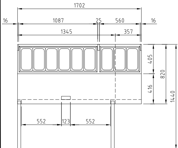
ВИД СВЕРХУ
