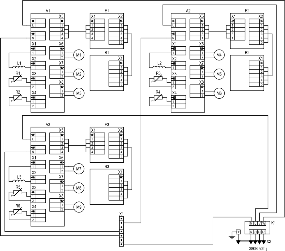
Схема индукционных плит комбо 700 и 900 серии, модели на 2 конфорки + однозонный гриль
