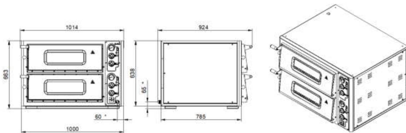
Рис. 1 - Общий вид печи ПЭП-4
