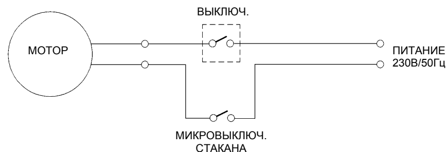
РИС. № 6 - Однофазная электрическая схема 230В
