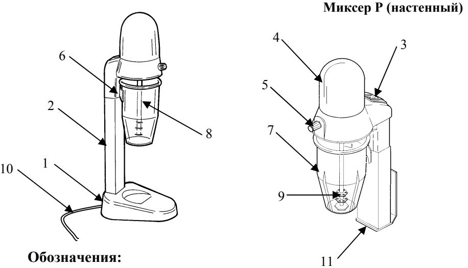
РИС. № 1 - Общий вид миксера
