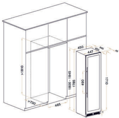
*Схема встройки в нишу.
