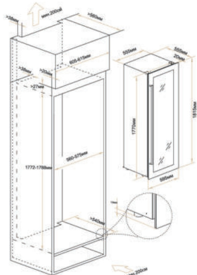
*Схема встройки в колонну.
