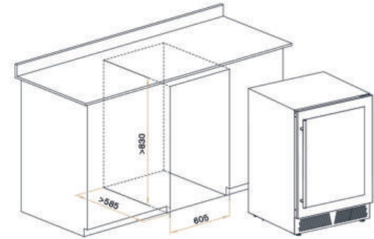
*Схема встройки под столешницу.
