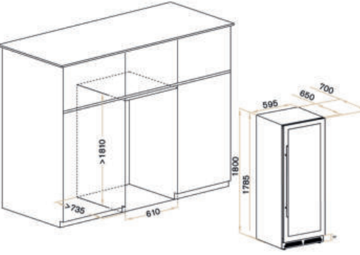
*Схема встройки в нишу.
