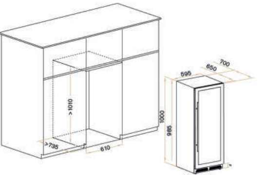
*Схема встройки в нишу.
