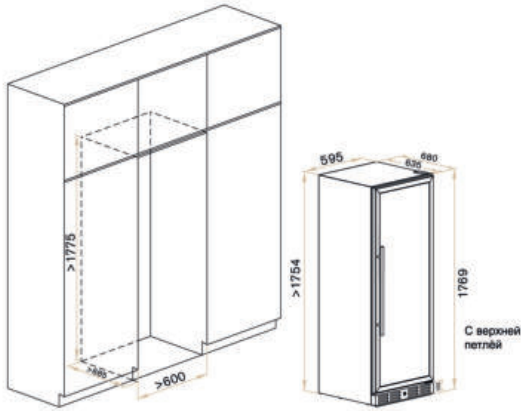
*Схема встройки в нишу.
