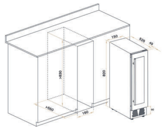
*Схема встройки под столешницу.
