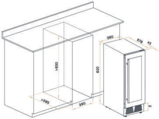
*Схема встройки под столешницу.
