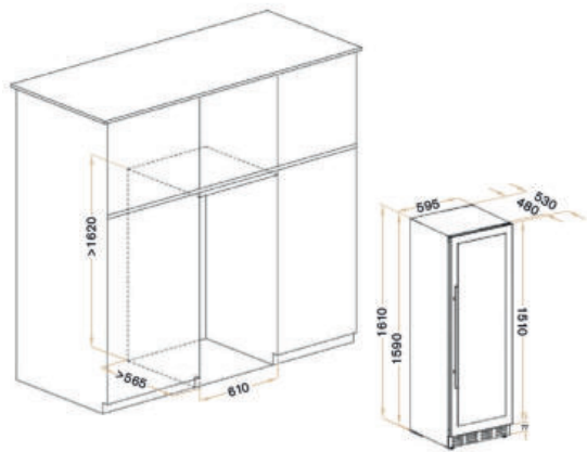
*Схема встройки в нишу.
