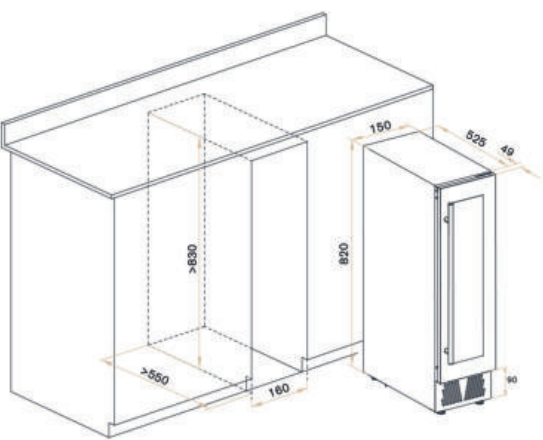
*Схема встройки под столешницу.
