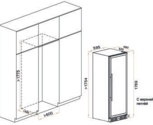
*Схема встройки в нишу.
