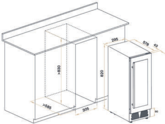
*Схема встройки под столешницу.
