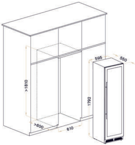
*Схема встройки в нишу.
