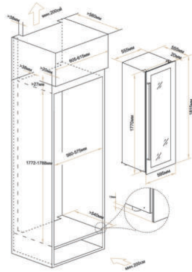
*Схема встройки в колонну.
