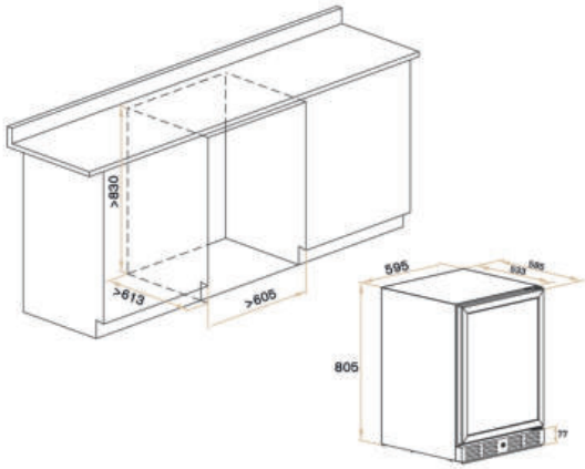
*Схема встройки под столешницу.
