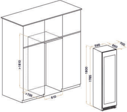
*Схема встройки в нишу.
