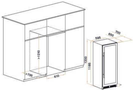
*Схема встройки в нишу.
