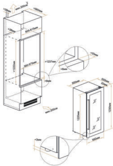
*Схема встройки в колонну.
