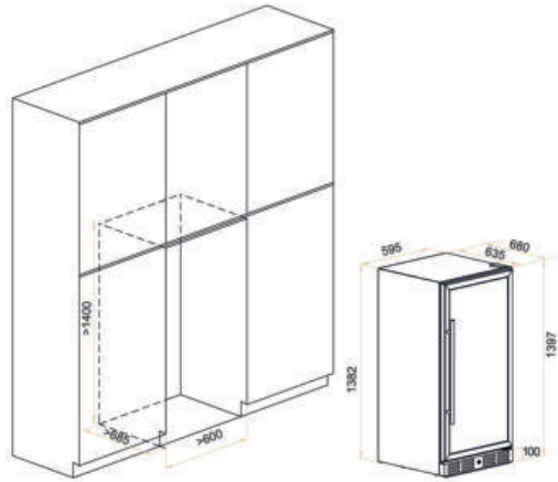
*Схема встройки в нишу.
