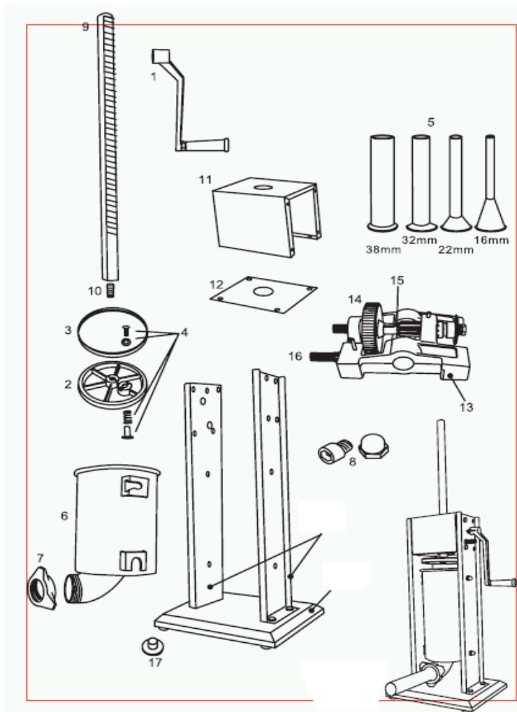
Рис1. Детализовка оборудования
