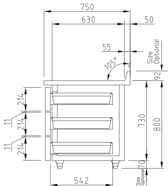
ВИД СБОКУ
