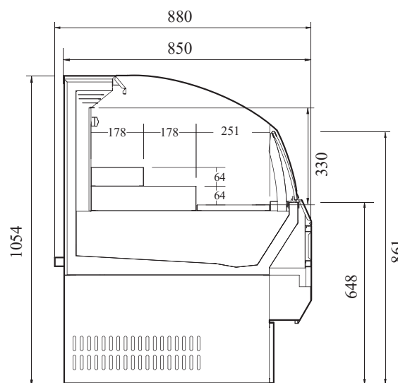
ВИД СБОКУ
