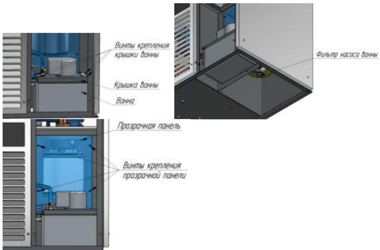
Рис. 6 Расположение крышки ванны, фильтра насоса и прозрачной панели. Смотровая панель на рис.6 не показана.
