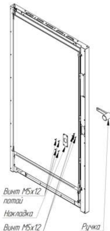
Рис. 10. Замена ручки
