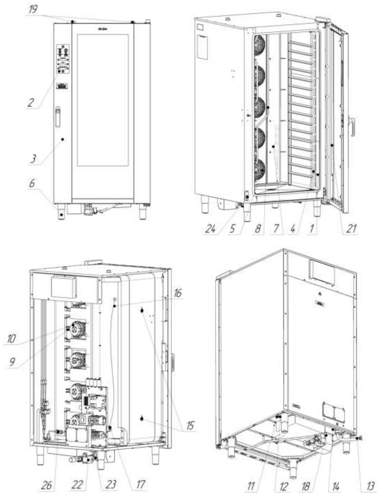
Рис. 16 Общий вид печи КЭП-16П
