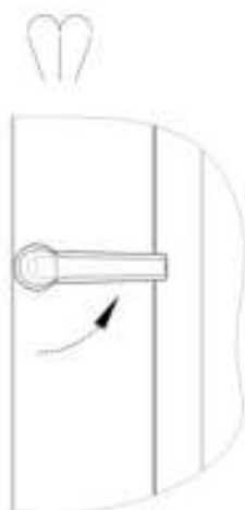
Рис. 6. Положение ручки двери при выпуске пара
