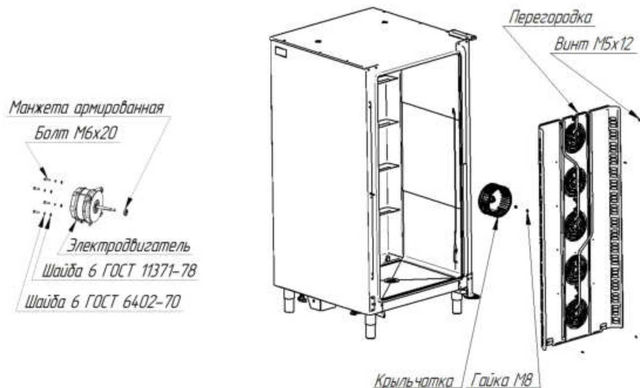
Рис. 11. Замена манжет
