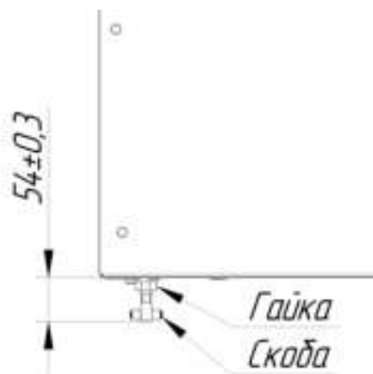
Рис. 13. Регулировка замкового устройства
