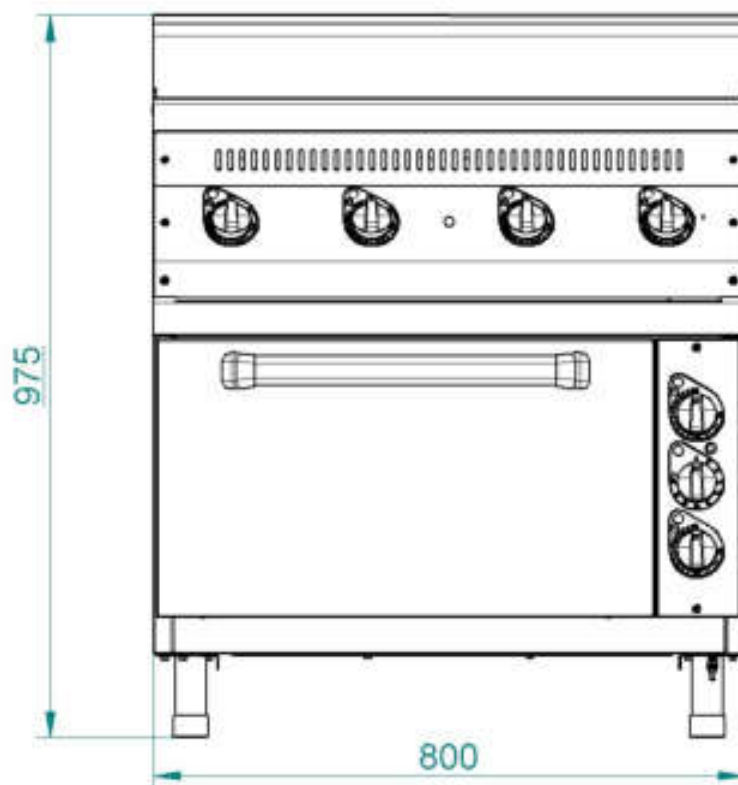
Рис. 11 Плита электрическая ЭПК-47ЖШ (вид спереди)
