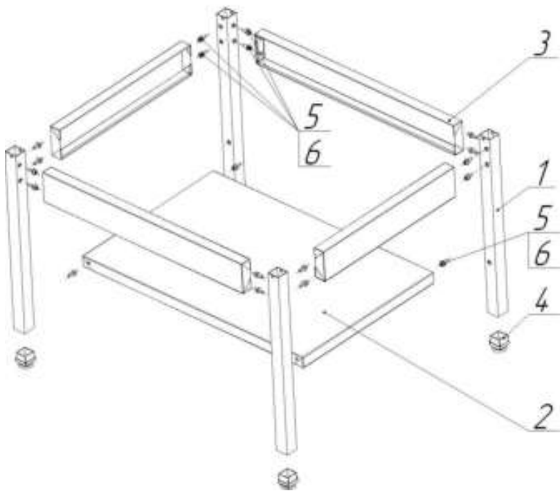
Рис.1: Сема сборки Подставки под ПКИ.
