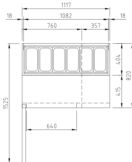
ВИД СВЕРХУ
