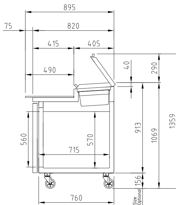
ВИД СБОКУ
