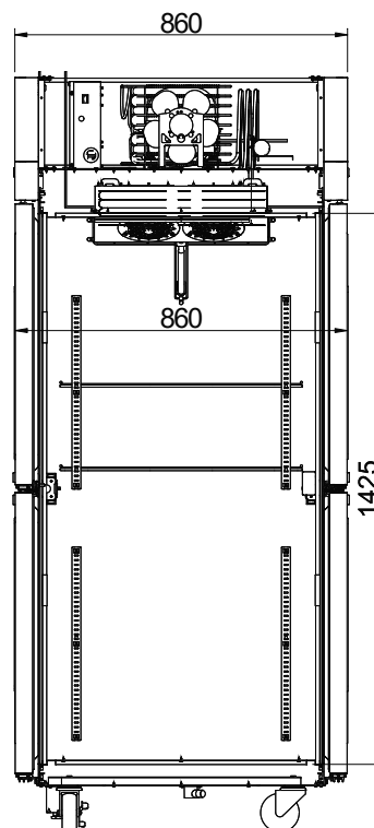
ВИД СБОКУ
