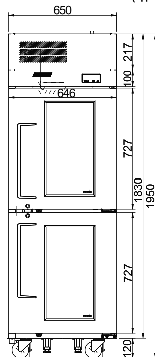
ВИД СПЕРЕДИ
