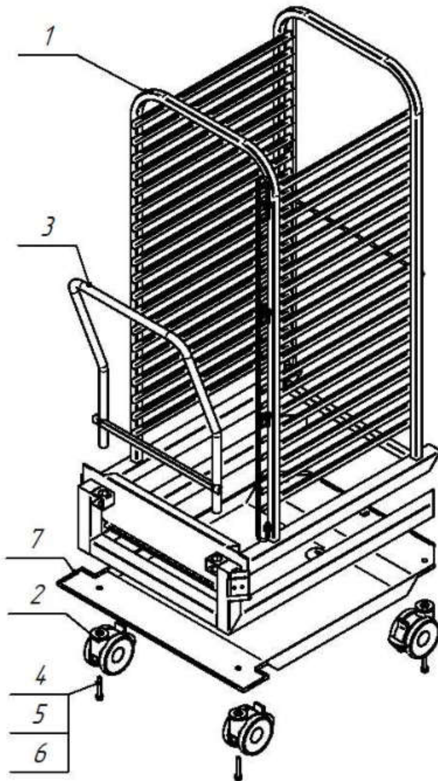
Рис. 1 Эскиз сборки тележки
