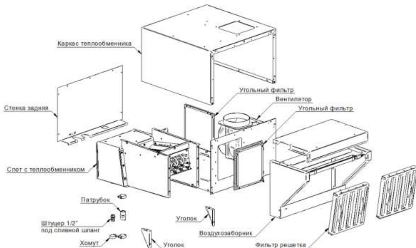
Рис 3 - Состав зонта
