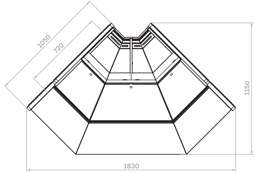
Внутренний угол (динамическое охлаждение)
