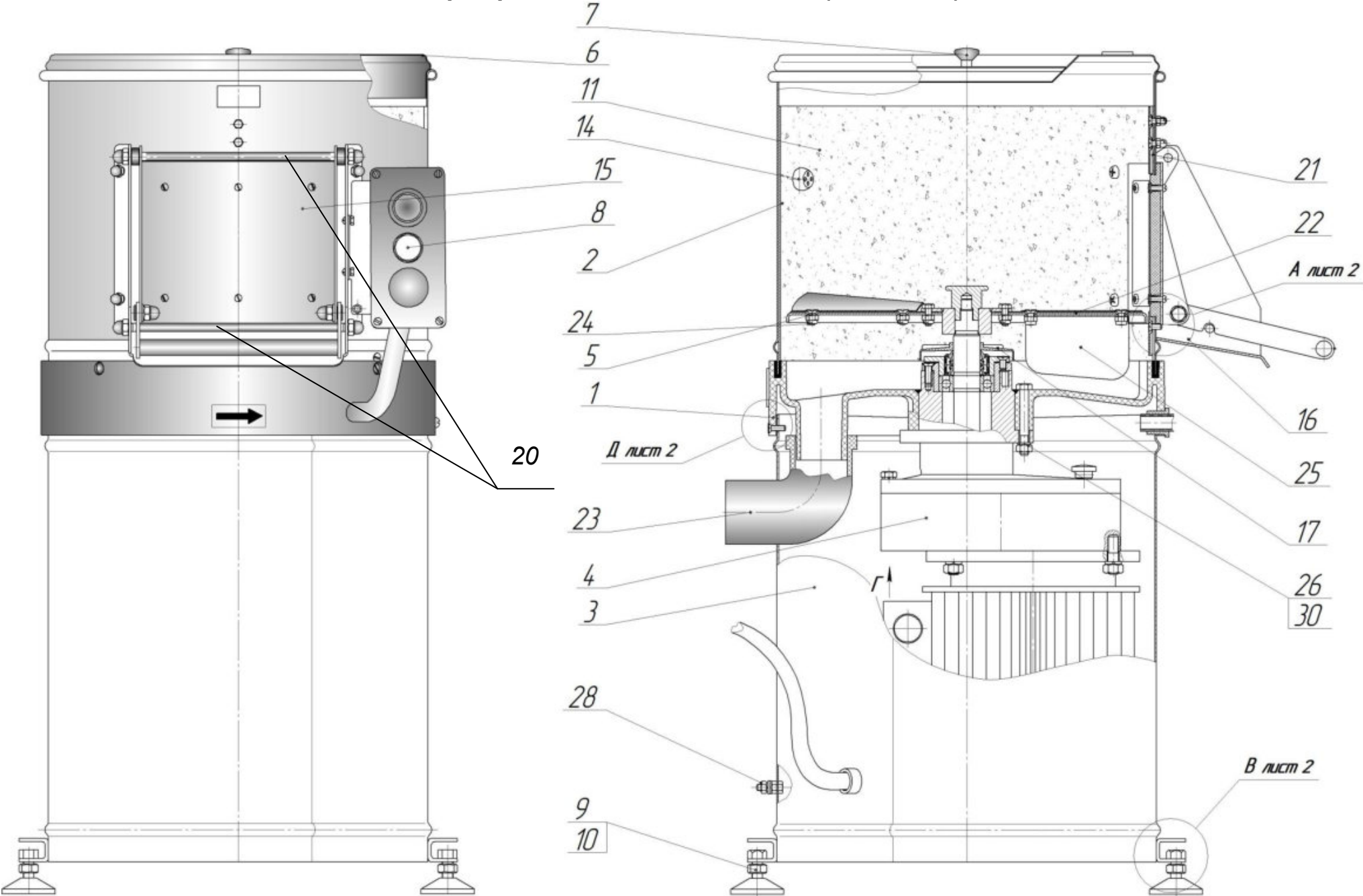
Машина картофелеочистительная К-150 (без литья), лист 1
