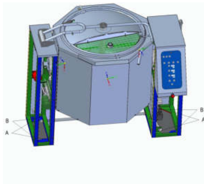
Рис. 4 Распаковка и установка котла
