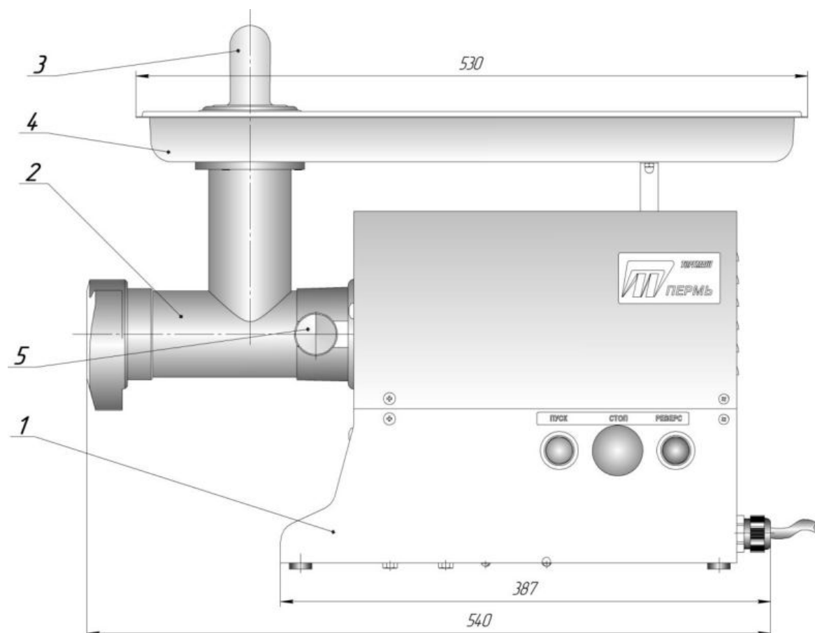
Рисунок 1 – Мясорубка М-150
