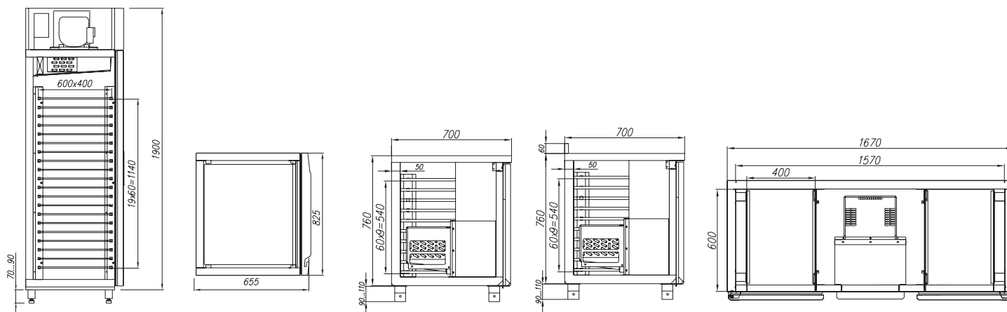
Шкаф M560
