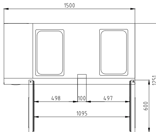
ВИД СВЕРХУ
