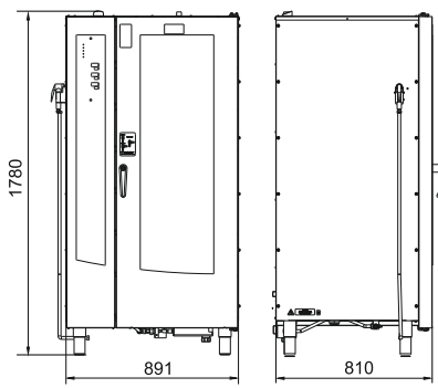
ПТП-20
