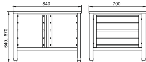
ЗВВ-800, ЗВВ-900
