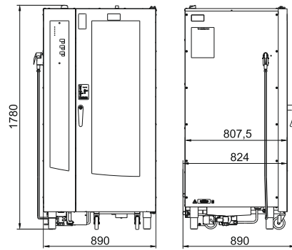
РКГ-6
