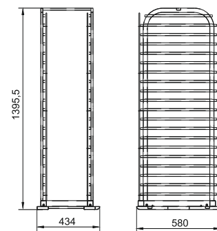
ШС-20-1/1
