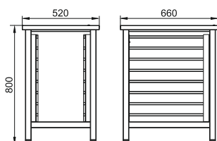
ПК-8-02
