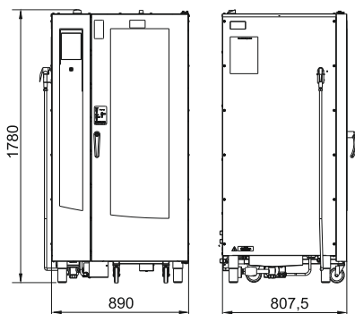
ШРТ 10-1/1М
