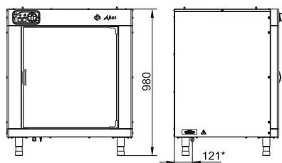
ПК-8-02
