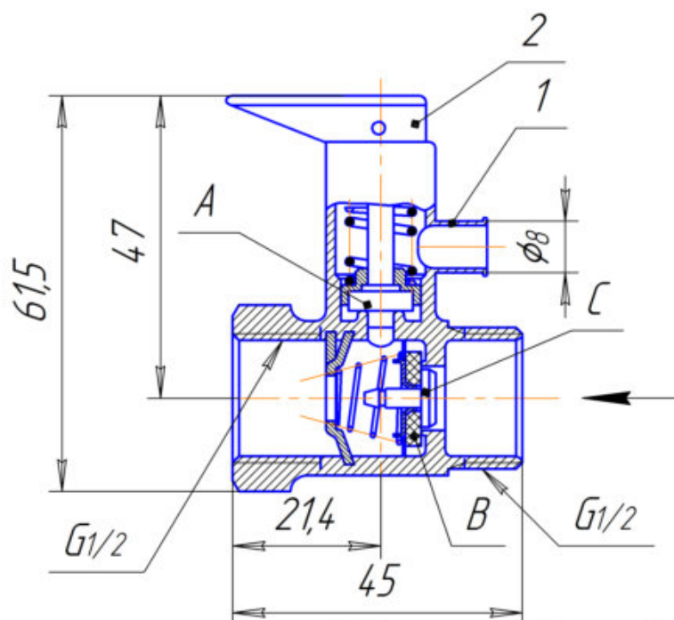
А - клапан предохранительный, В - клапан обратный, С - клапан перелива, 1 - отверстие переливное, 2 - рычаг
