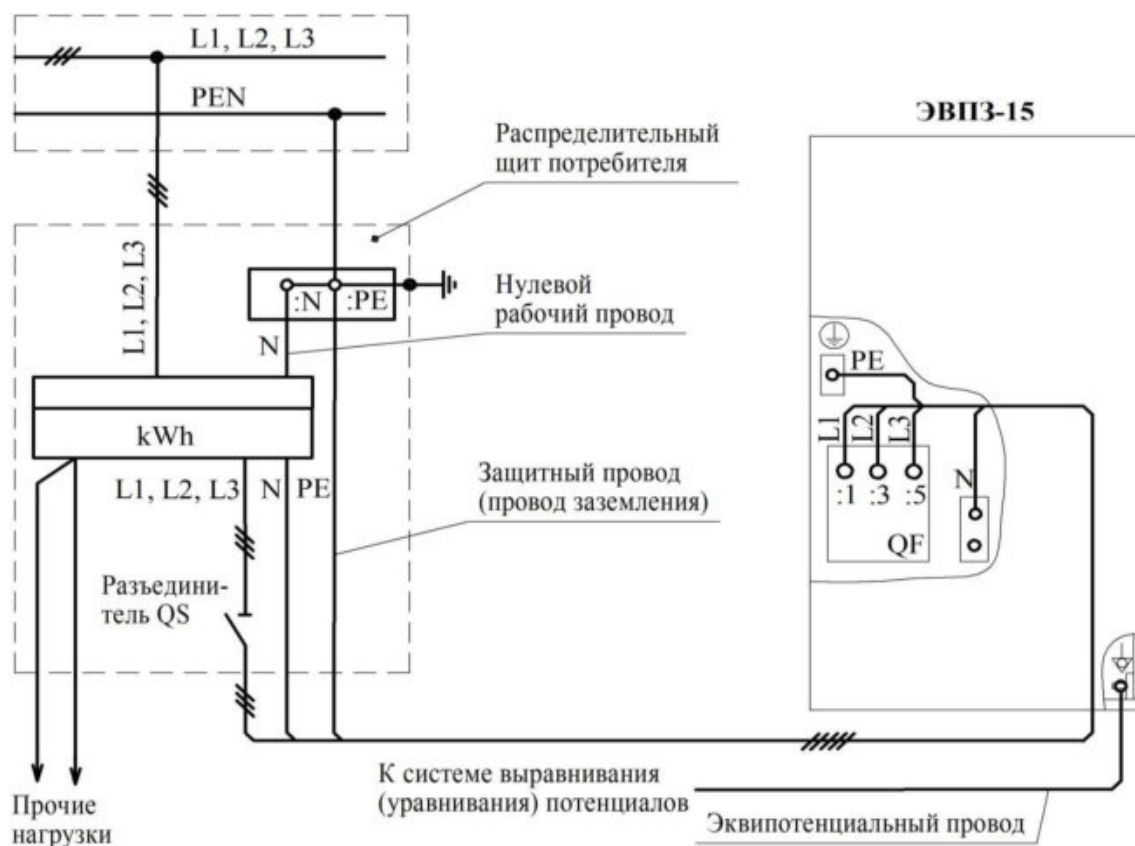
Рисунок 6 – Схема подключения водонагревателя ЭВПЗ-15 к электросети
