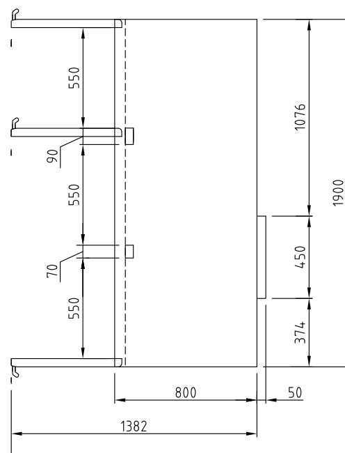
ВИД СВЕРХУ
