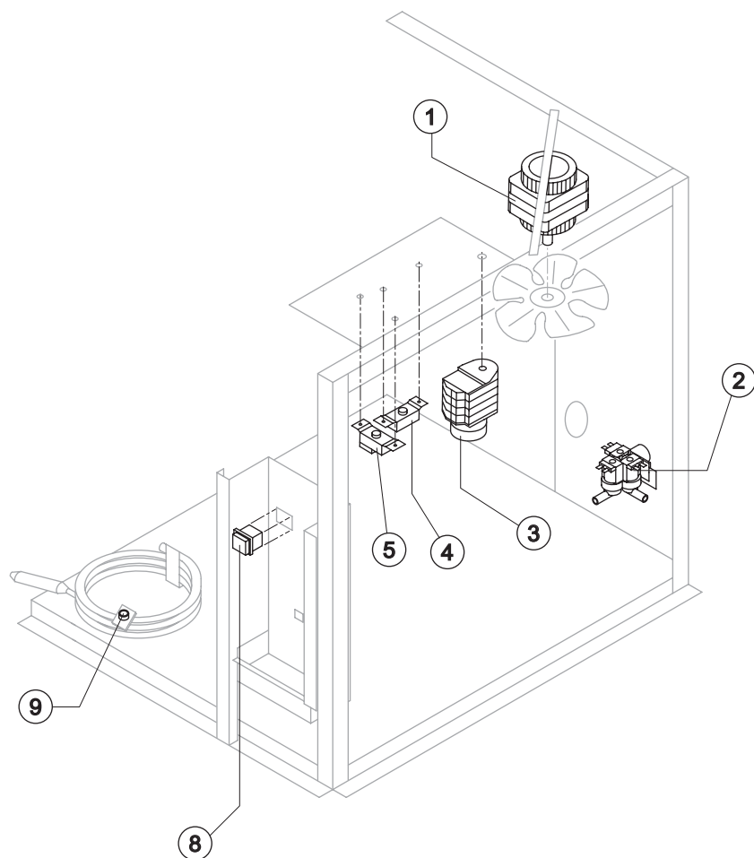
Ref. 1 - Fan Motor
