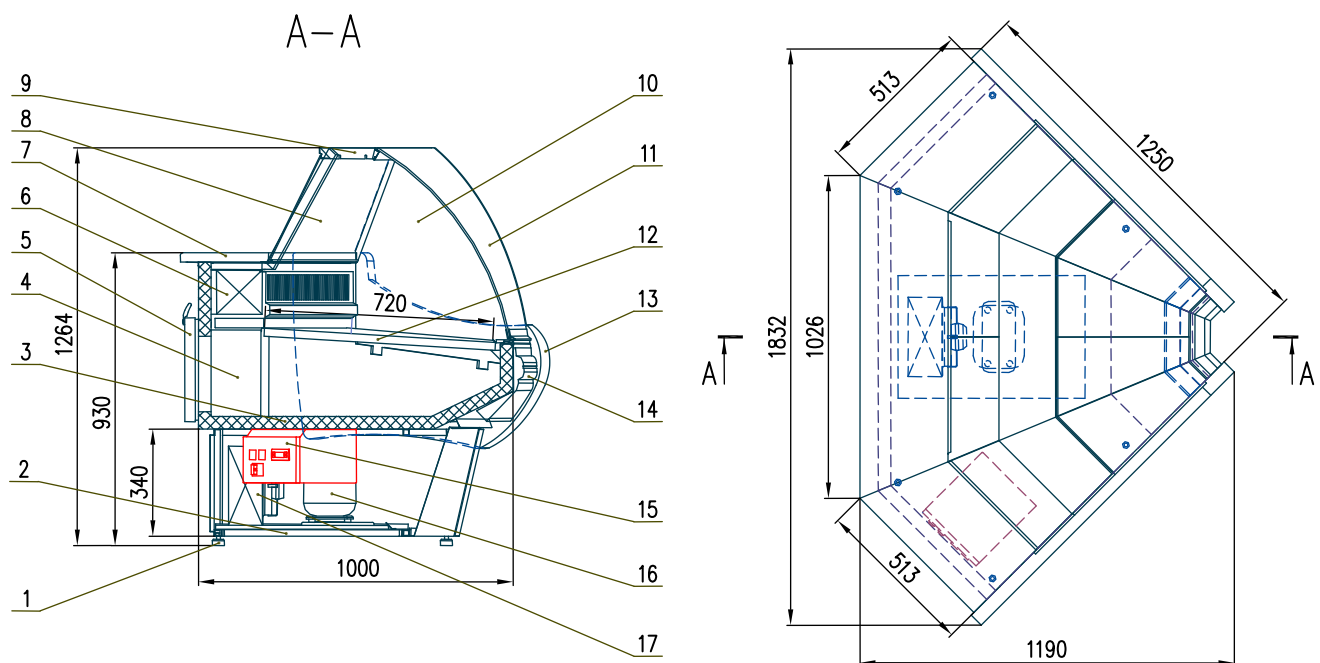
Рис. 16. Схема витрины «ВИЛИЯ» УВ 90 ВС
