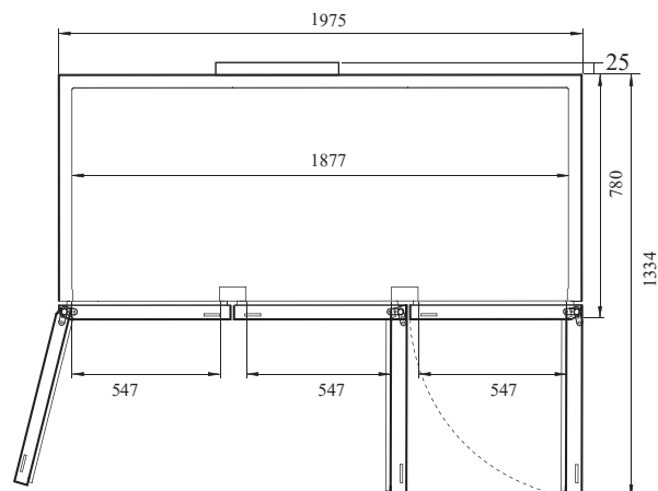
ВИД СВЕРХУ
