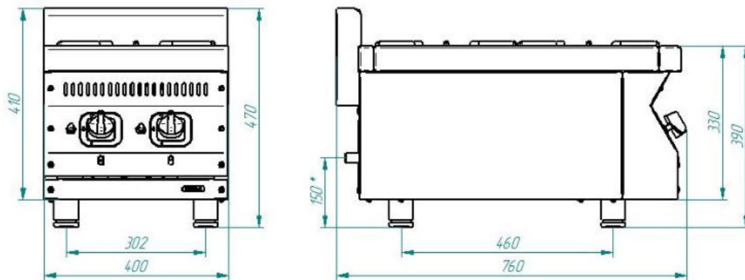
Габаритные размеры Газовой плиты ПГК-27Н-01-П-А
