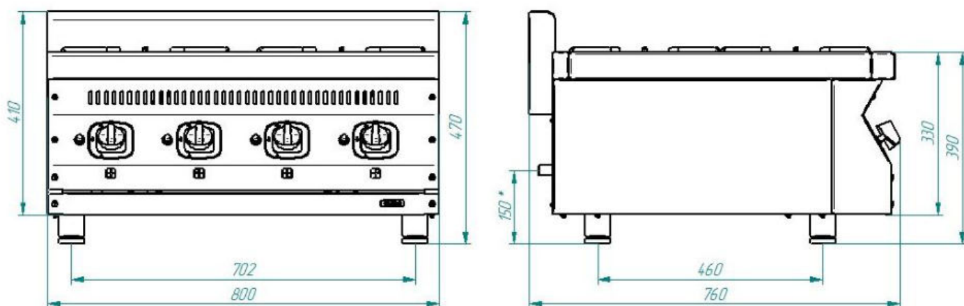
Габаритные размеры газовой плиты ПГК-47Н-01-П-А
