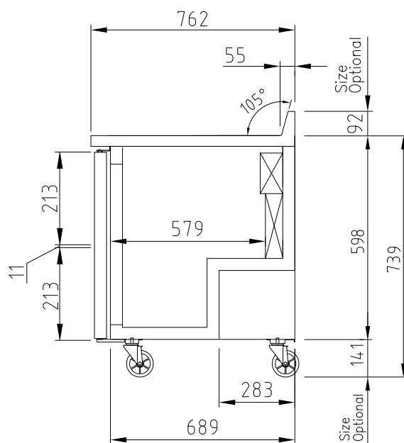
ВИД СБОКУ
