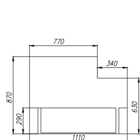
НЕЙТРАЛЬНЫЙ ПРИЛАВОК
