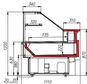
ХЛЕБНАЯ (НЕОХЛАЖДАЕМАЯ)
