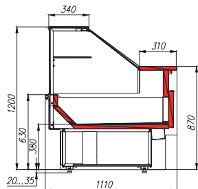
НЕЙТРАЛЬНЫЙ ПРИЛАВОК
