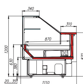
ВЕНТИЛИРУЕМАЯ (ДИНАМИКА)
