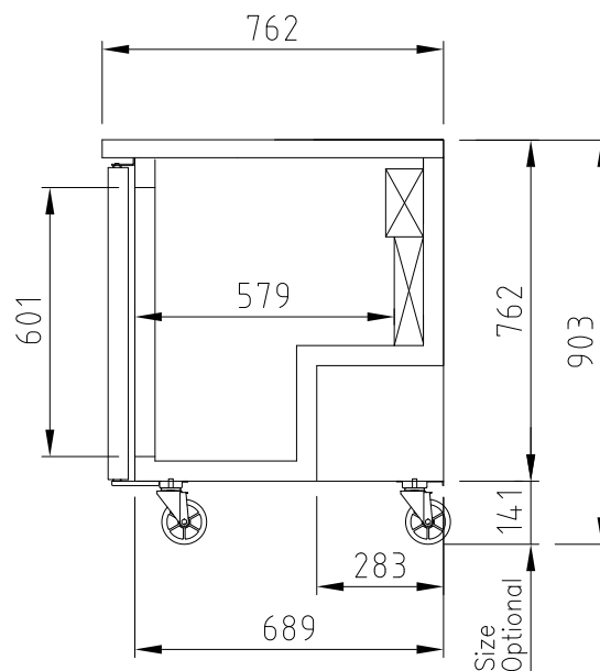
ВИД СБОКУ
