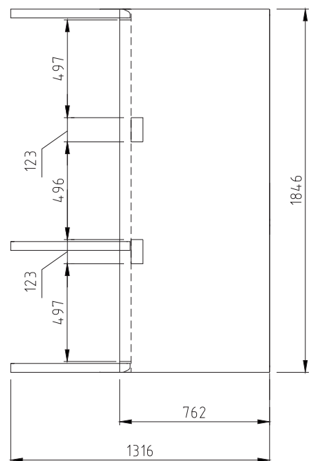
ВИД СВЕРХУ
