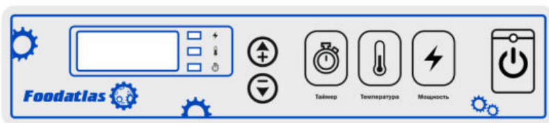
Рис №3 Панель управления для моделей Плита индукционная Foodatlas FA-3500 Eco Плита индукционная Foodatlas FA-3500W Eco Плита индукционная Foodatlas FA-35002H
