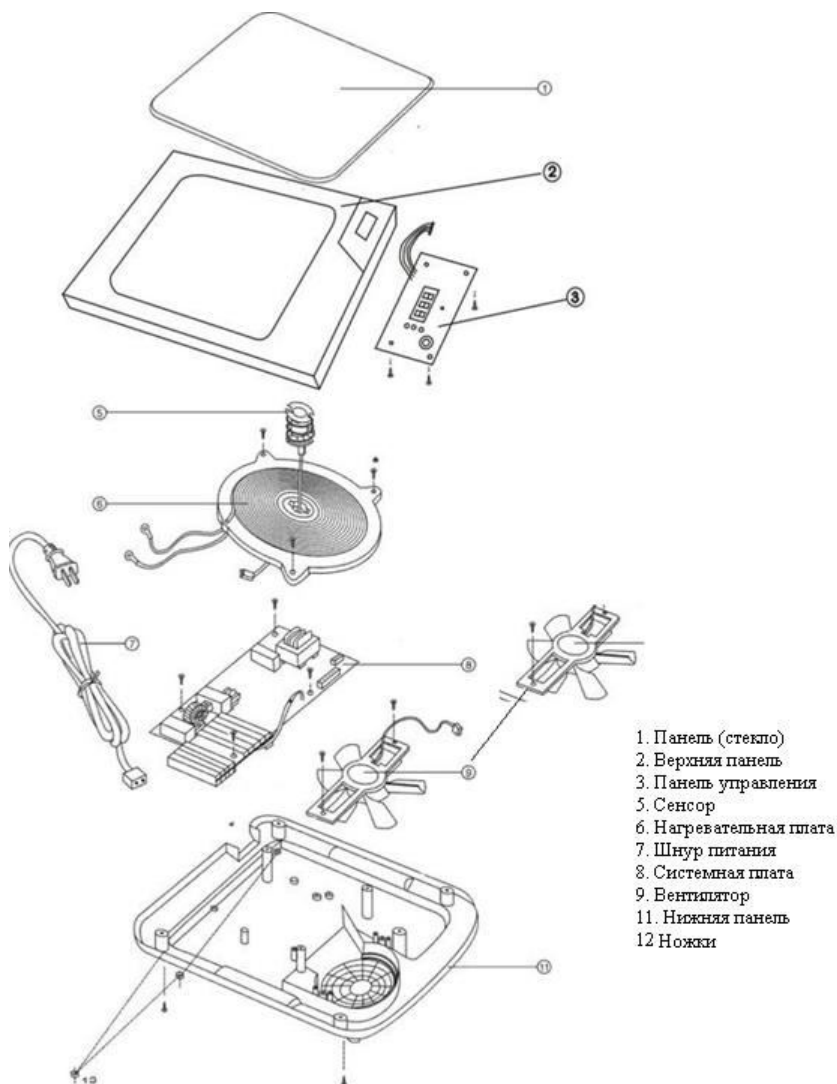
Рис. 4 Основные элементы оборудования для индукционной плиты с 1-ой рабочей поверхностью.
