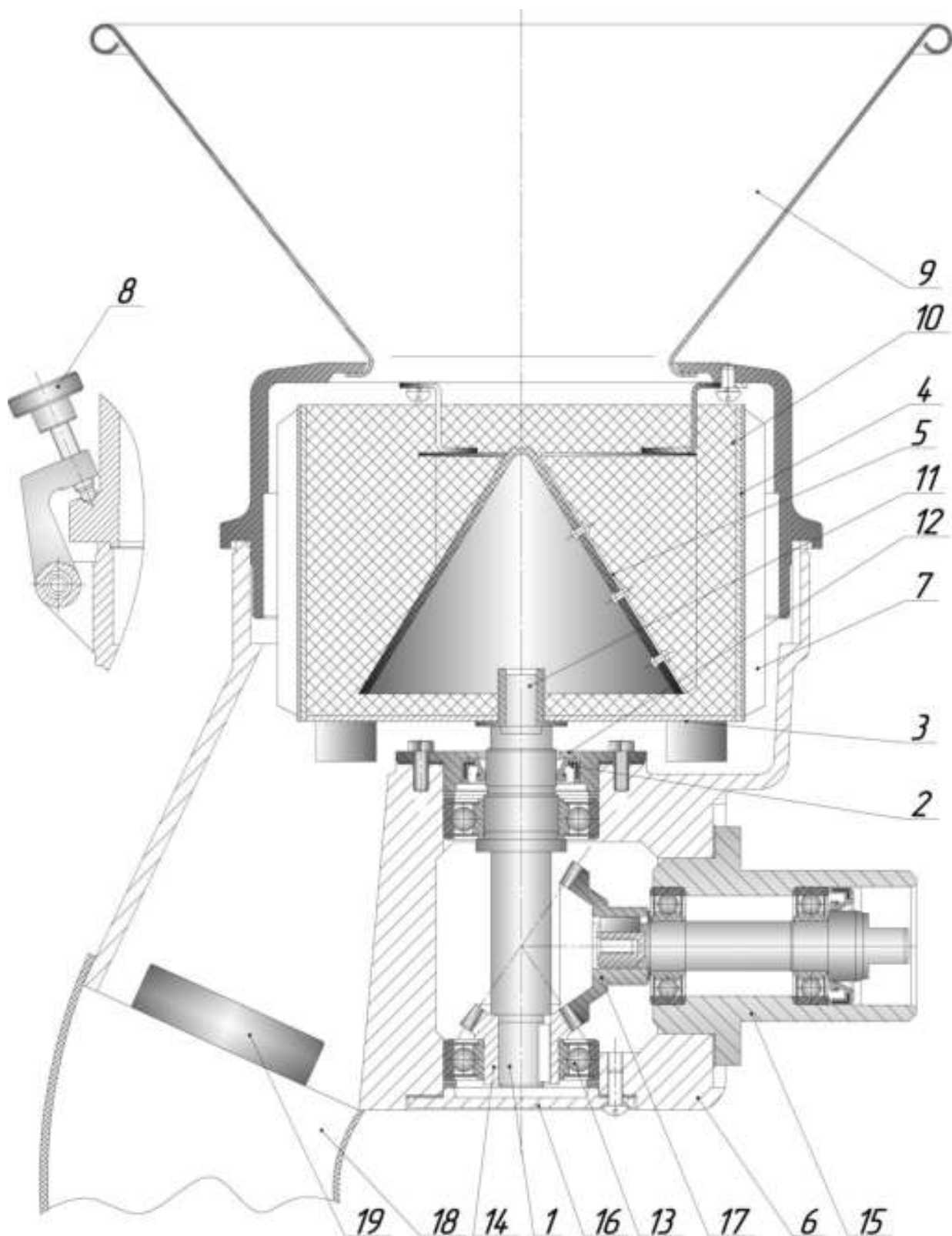
Рисунок 19 – Просеиватель МП – 01
