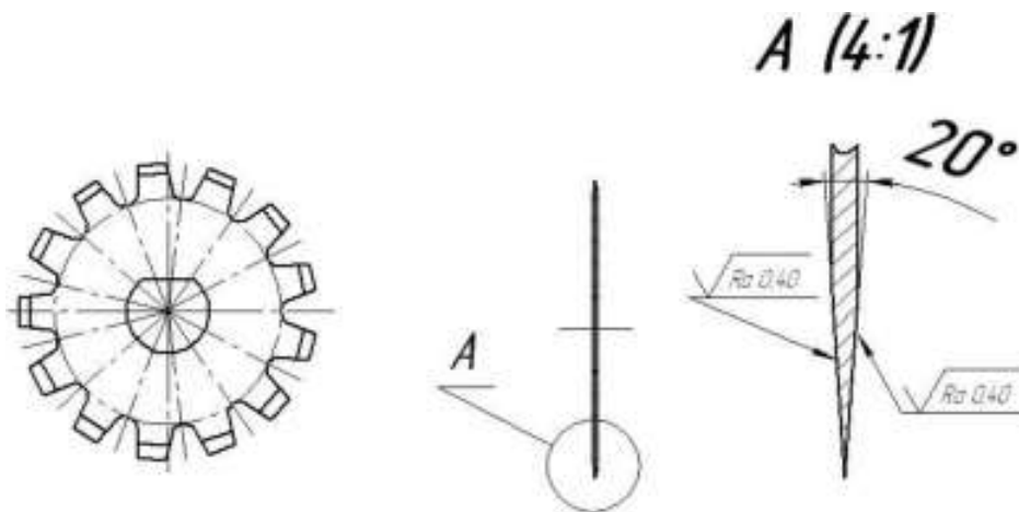
Рисунок – 22 Фреза
