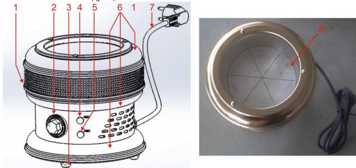
Рисунок 2: Компоненты прибора
