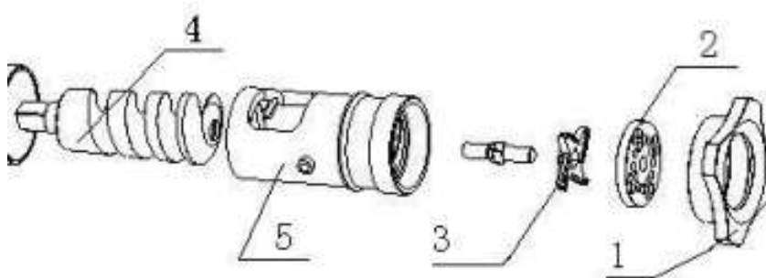
1-Шпонка 2-диск 3-лезвие 4-спираль 5-блок мясорубки
