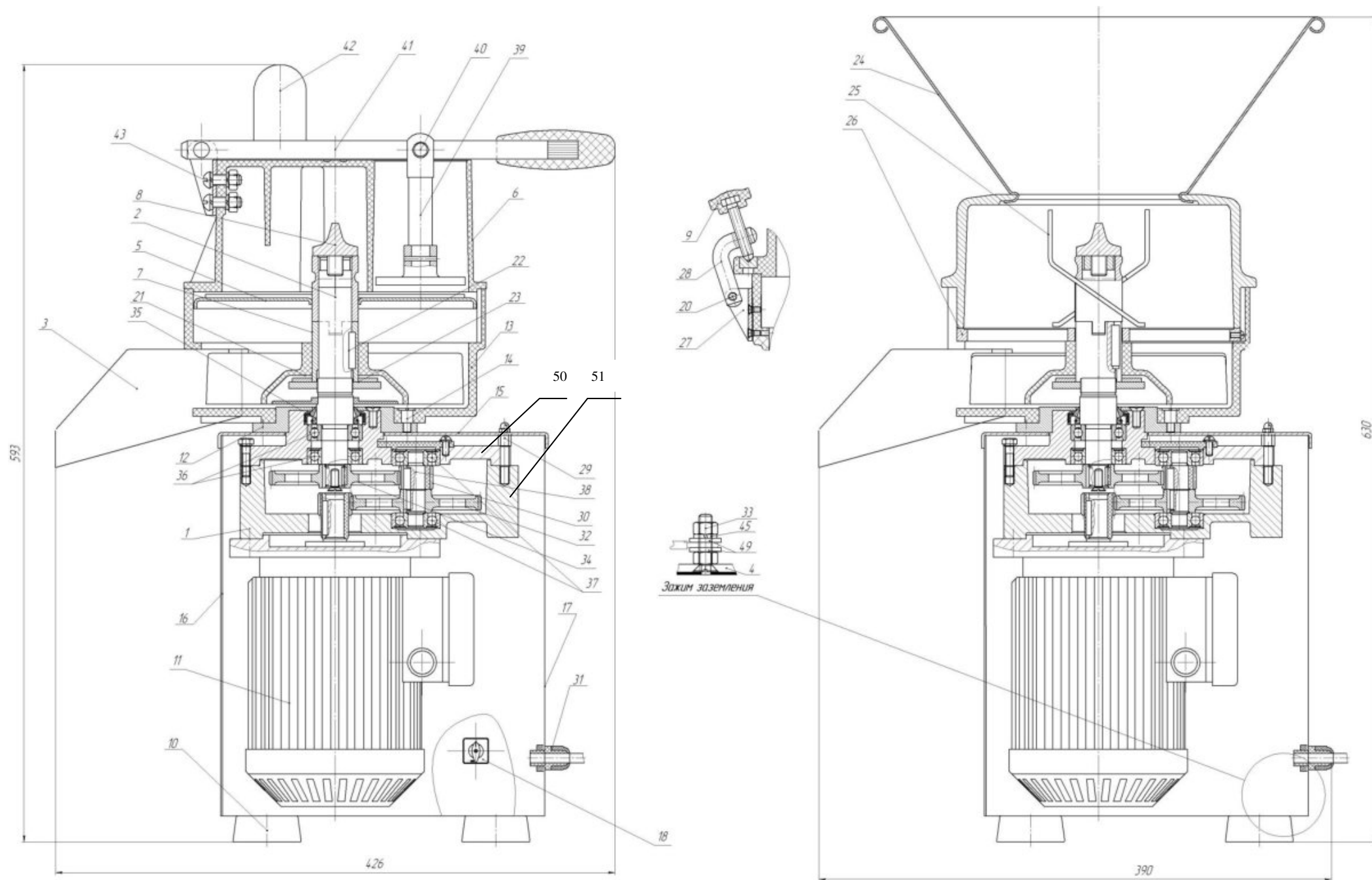
Машина овощерезательно-протирочная ОМ-350М
