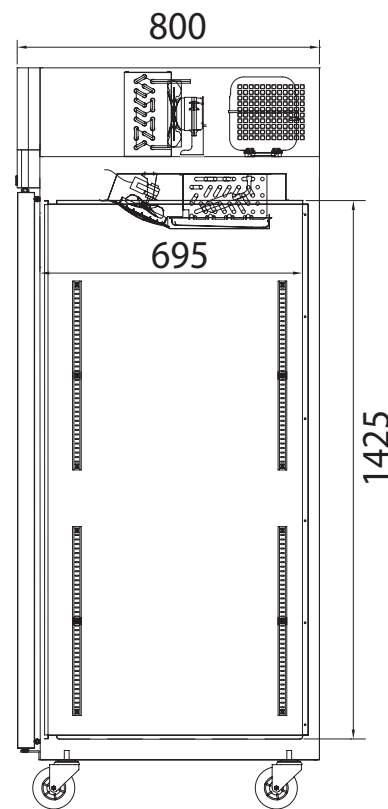
ВИД СБОКУ
