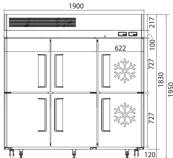
ВИД СПЕРЕДИ
