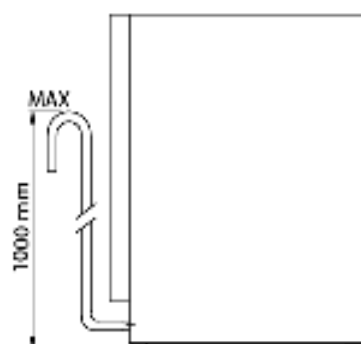
DRAIN PUMP MODELS MODELLI POMPA SCARICO ABLAUFpumpe Modelle MODELES POMPE DE VIDANGE MODELO DE BOMBA DE DRENAJE
