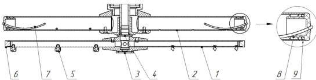
Рис.7. Схема установки разбрызгивателей
